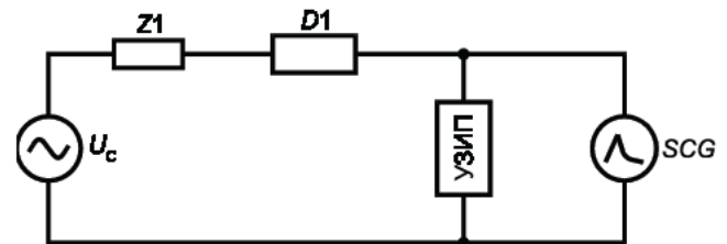
Рисунок 6а — Цепь для испытания УЗИП с сопровождающим током I_{\Pi} ниже заявленной способности выдерживать ток короткого замыкания
