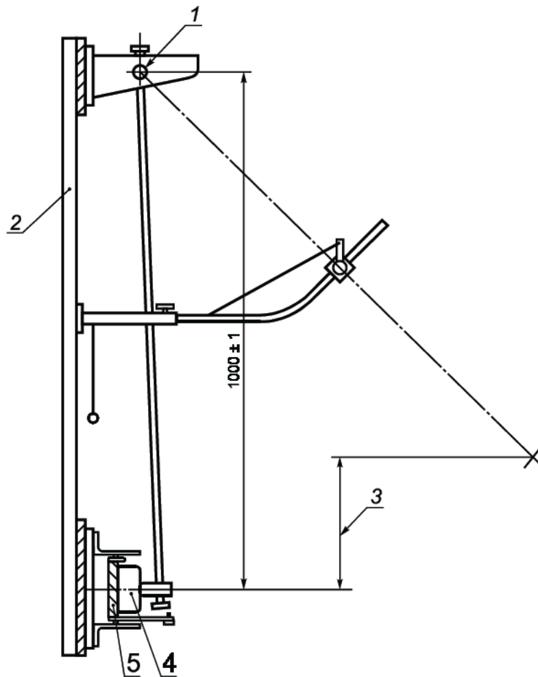
Рисунок 10а — Испытательная установка
